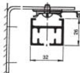
Zidna montaža s kutnicama za montažu i steznim zaporom. Savitljivo do promjera 350 mm
