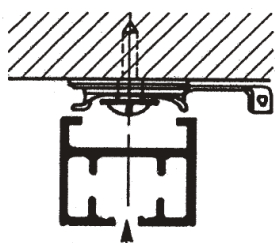
Stropna montaža sa steznim zaporom. Savitljivo do promjera 350 mm
