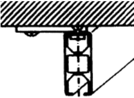
Stropna montaža 1 vod. sa nosačem AL0487K
