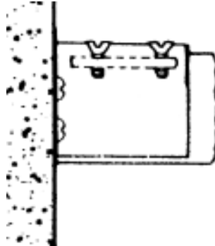
Zidna montaža 1 vod. sa nosačem AL0481K
